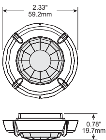
FSP-L2 dimensions
