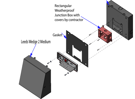
SCBT Surface Conduit Box Trim
